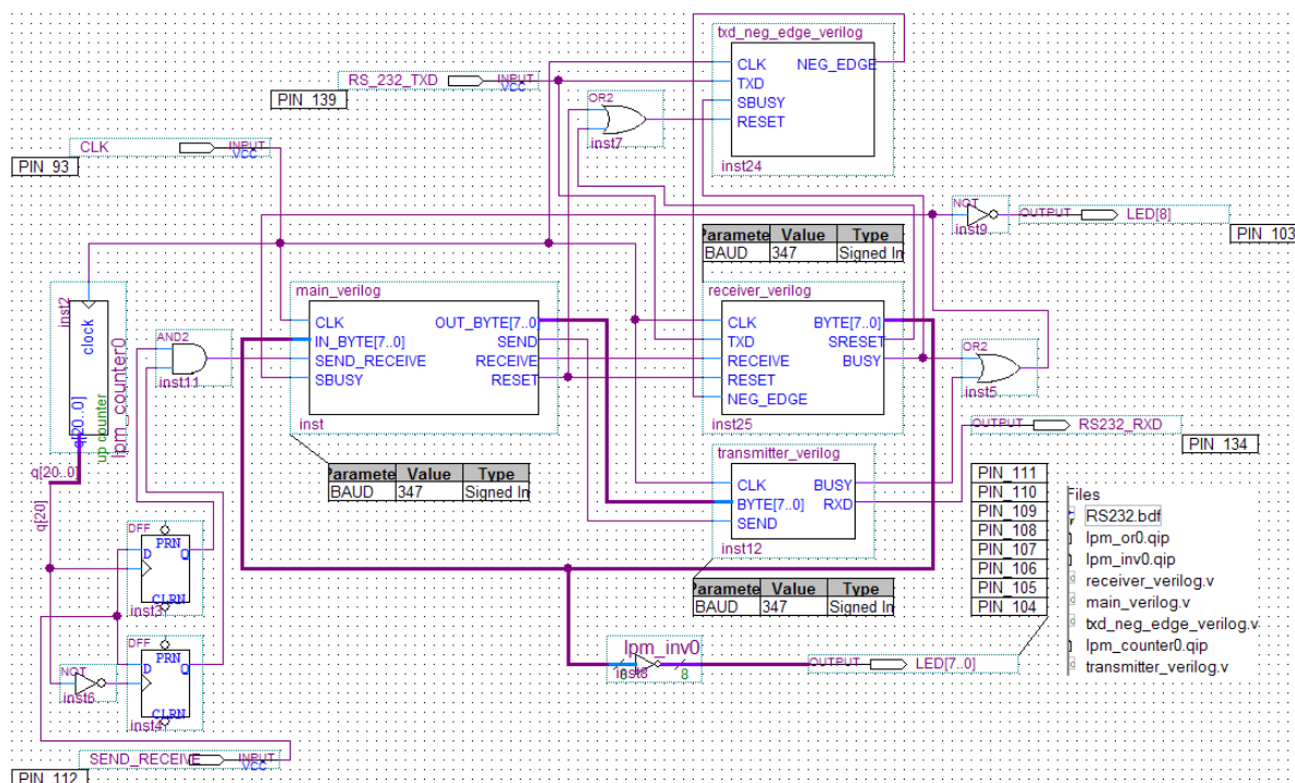
Рис. 2. Структурно-функциональная схема устройства работы с последовательным портом
