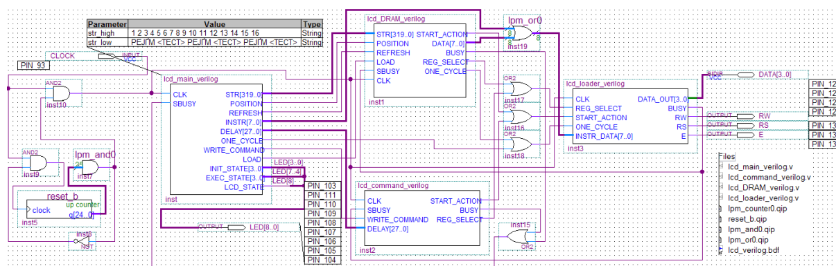
Рис.1. Структурно-функциональная схема устройства управления дисплеем
