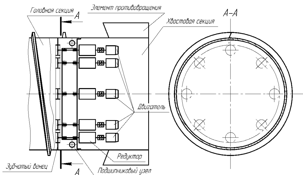
Рис. 4. Кинематическая схема трансмиссии геолода с многопоточным редукторным приводом
