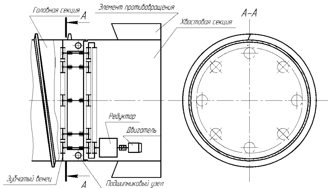
Рис. 3. Кинематическая схема трансмиссии геолода с редукторным приводом с многопоточной выходной ступенью
