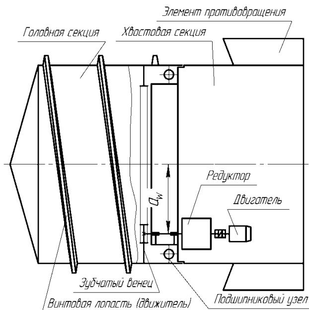
Рис. 1. Кинематическая схема трансмиссии геогода с редукторным приводом
