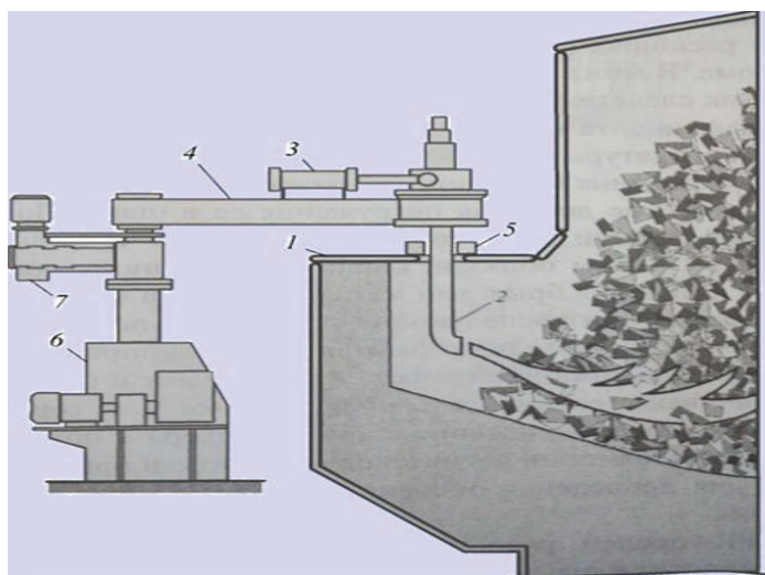
Рис. 4. Установка HPR-горелки в дополнительном эркере: 1 – водоохлаждаемая крышка; 2 – горелка; 3 – цилиндр; 4 – кронштейн; 5 – уплотнитель; 6 – механизм подъема установки; 7 – механизм отвода горелки
