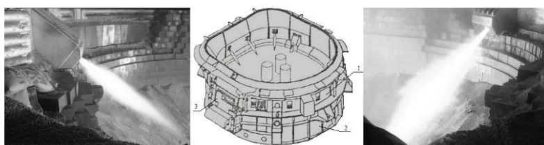
Рис. 1. Топливно-кислородные горелки в ДСП
