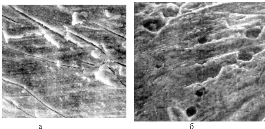
Рис. 1. Микротрещины (а) и кратеры (б) на поверхности титана после 120 мин наводороживания (увеличение 1500)
