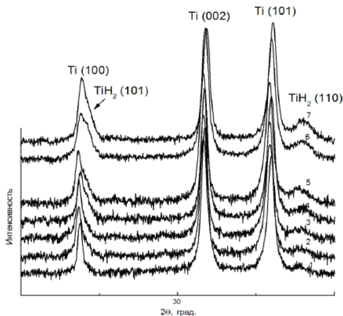
Рис. 3. Динамика образования фазы TiH 2
