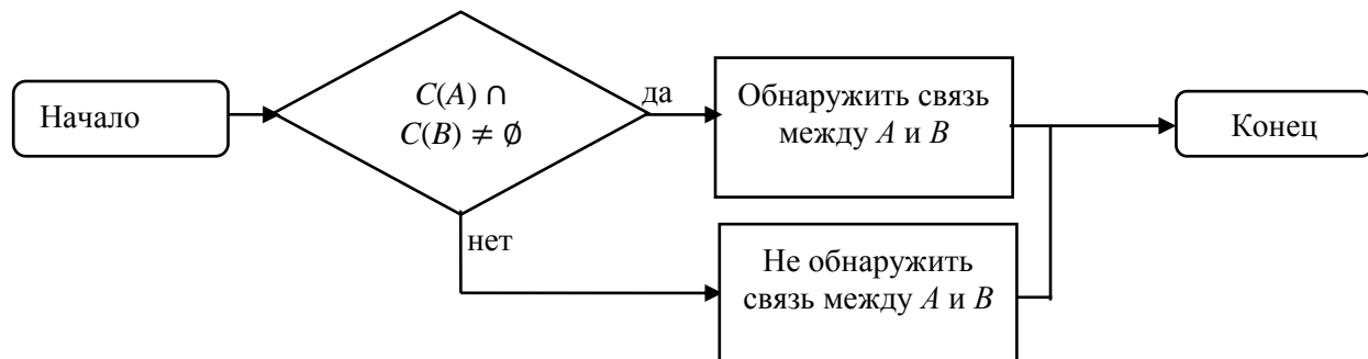
Рис. 1. Алгоритм определения возможности получения логических выводов из двух вершин
