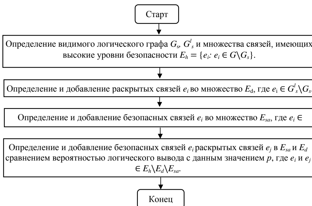
Рис. 3. Алгоритм обнаружения нарушения логических выводов
