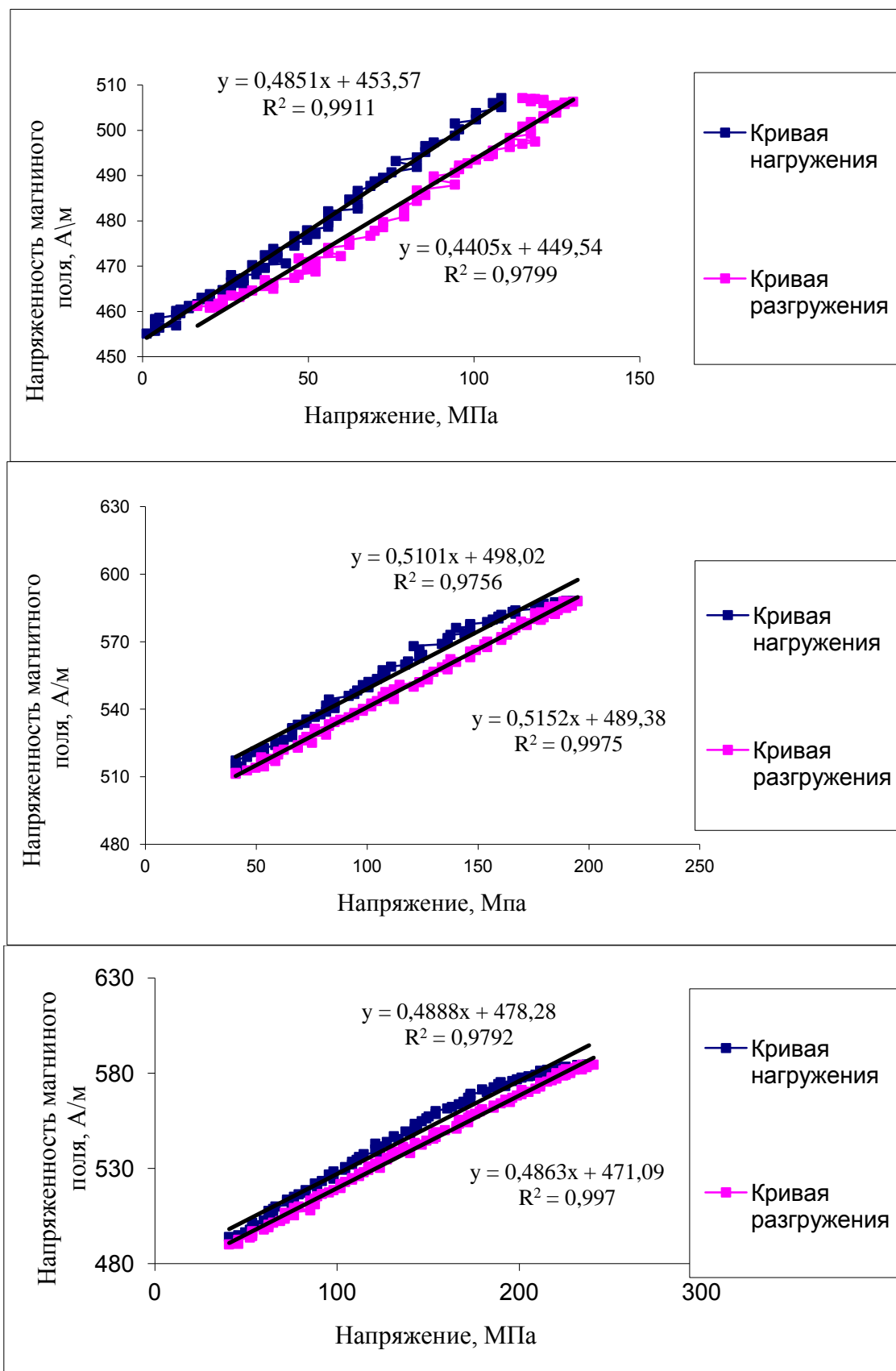
Рис. 3. Построение линий тренда по кривым нагружения и разгружения
