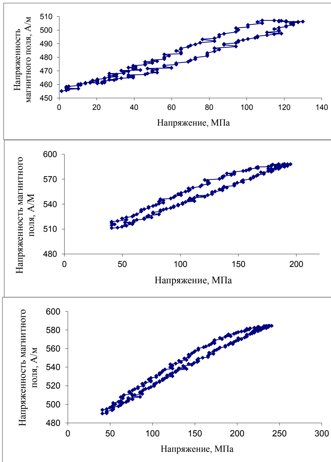
Рис. 2. Связь между величиной механического напряжения и напряженностью магнитного поля рассеяния для образца K40, отпущенного при температуре 600 °С
