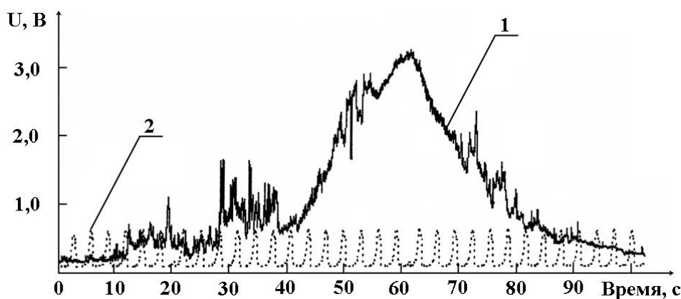
Рис. 2. Сигнал на выходе блока акустического датчика в момент прохождения очистного устройства типа СКР-3: 1 – сигнал очистного устройства; 2 – калибровочный сигнал, равный по амплитуде порогу срабатывания СПРА-4
