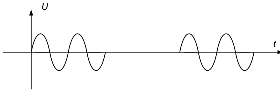
Рис. 2. Форма сигнала для получения субгармонических составляющих
