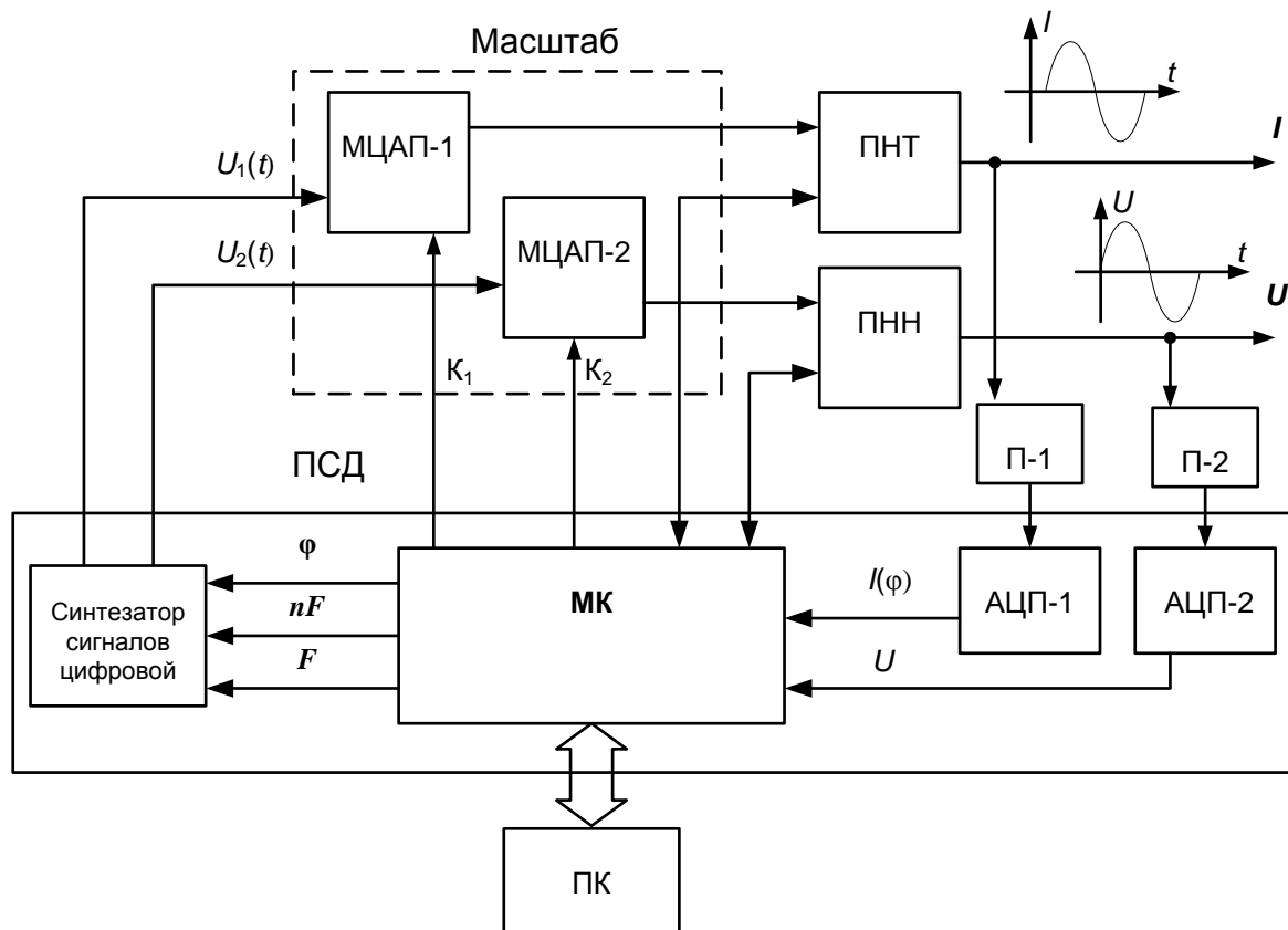
Рис. 3. Функциональная схема КФМ с обратной связью по мгновенному значению и автоматической коррекцией погрешности
