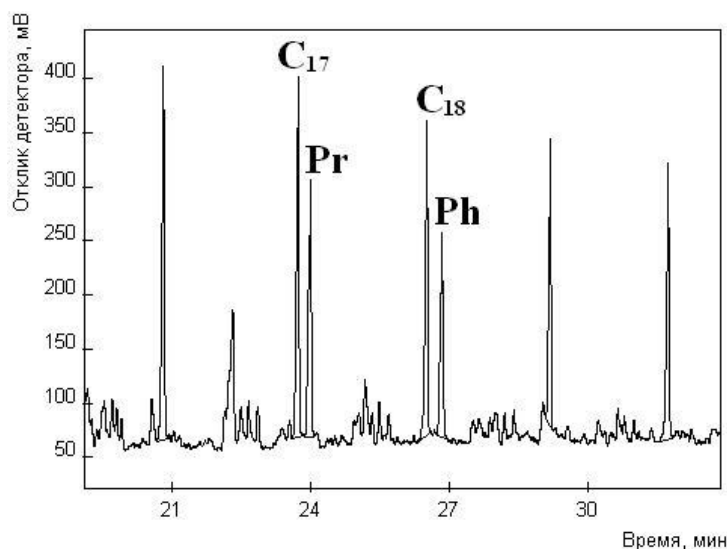
Рис. 1. Хроматограмма масляной фракции нефти из почвы на 30-е сутки биодegradации почвенной микрофлорой
