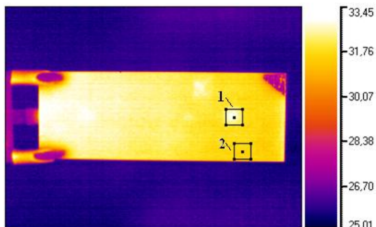
Рис. 2. Исходная последовательность ИК-термограмм в виде матрицы размером 240 \times 320 \times 501
