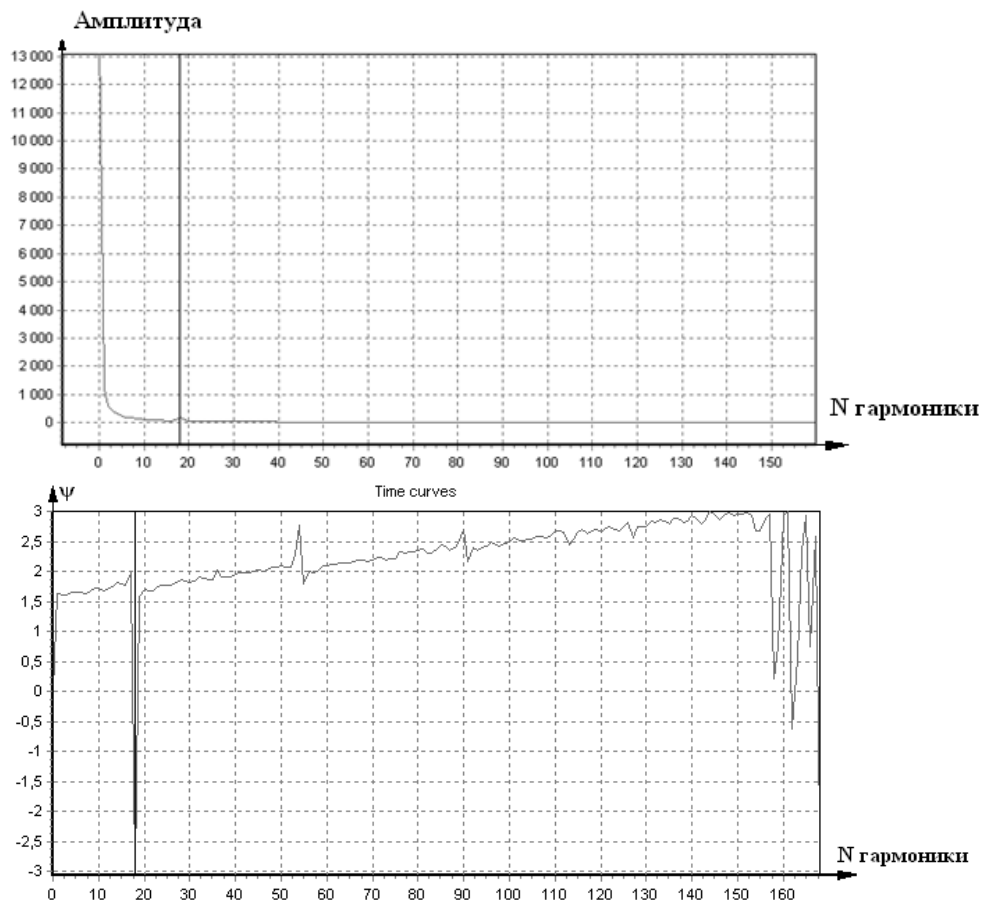
Рис. 6. Амплитудный и фазовый спектры преобразования Фурье
