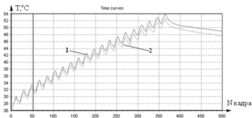
Рис. 3. Изменение средней температуры в дефектной и бездефектной зонах
