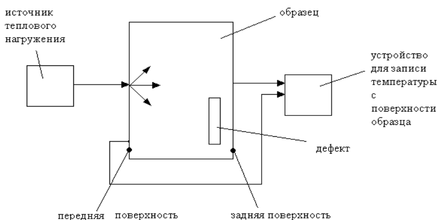
Рис. 1. Общая схема активного теплового контроля [3]
