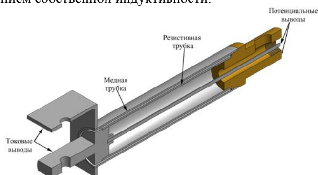
Рис. 1. Конструкция коаксиального шунта
