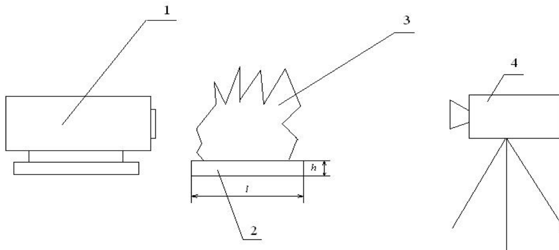
Рис. 1. Схема экспериментальной установки: 1 – модель АЧТ-45/100/1100; 2 – слой исследуемого материала с длиной l и высотой h ; 3 – пламя фронта горения; 4 – спектрограф SOLAR III MS2001i
