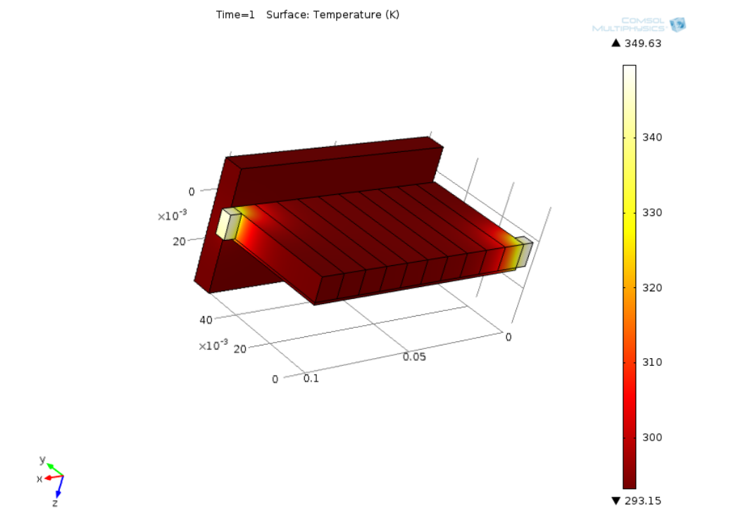
Рис. 3. Распределение температурного поля в пакете пластин, закрепленном на теплоотводе Т-образного сечения
